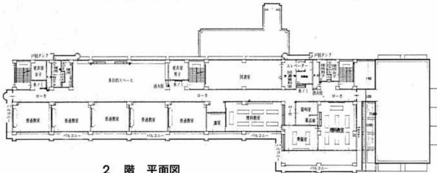
2階平面図
