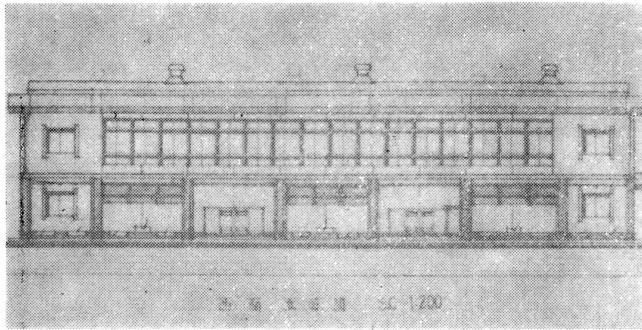
写真 上 北面立面図 右上 南面立面図 下 西面立面図 右下 東面立面図
