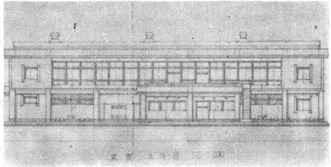
写真 上 北面立面図 右上 南面立面図 下 西面立面図 右下 東面立面図
