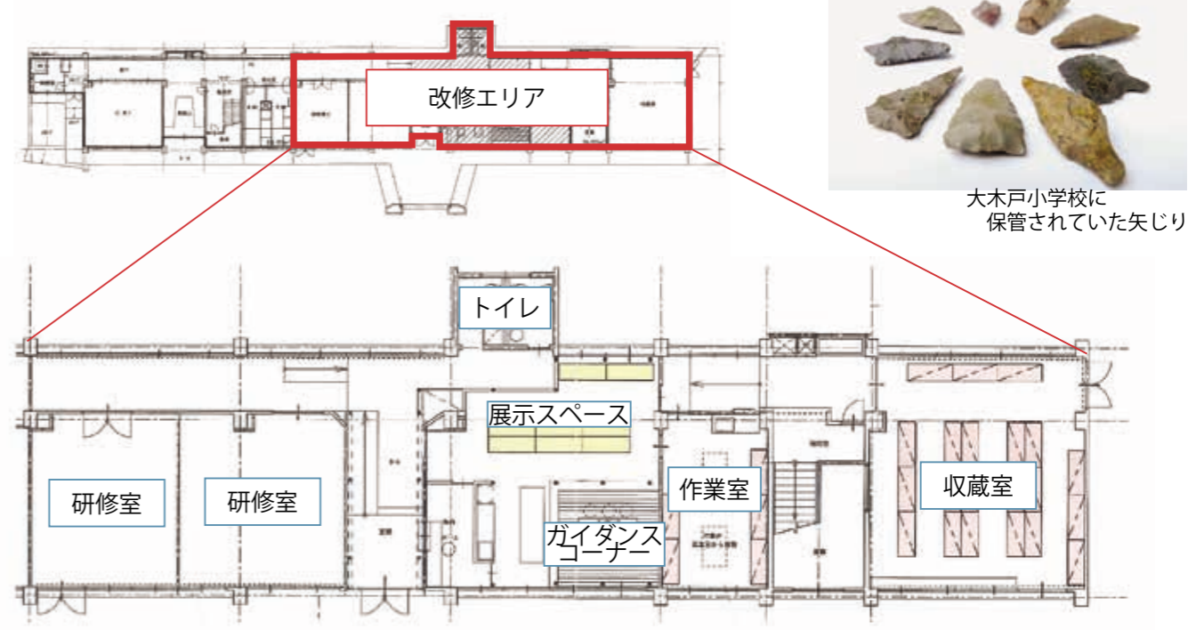
【校舎 1 階部分平面図】
