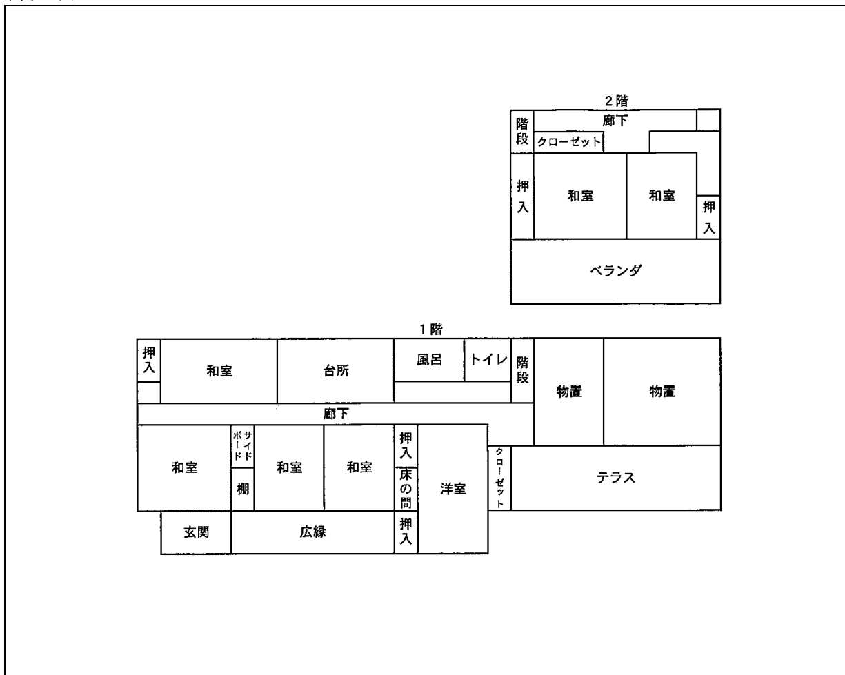
間取り図
